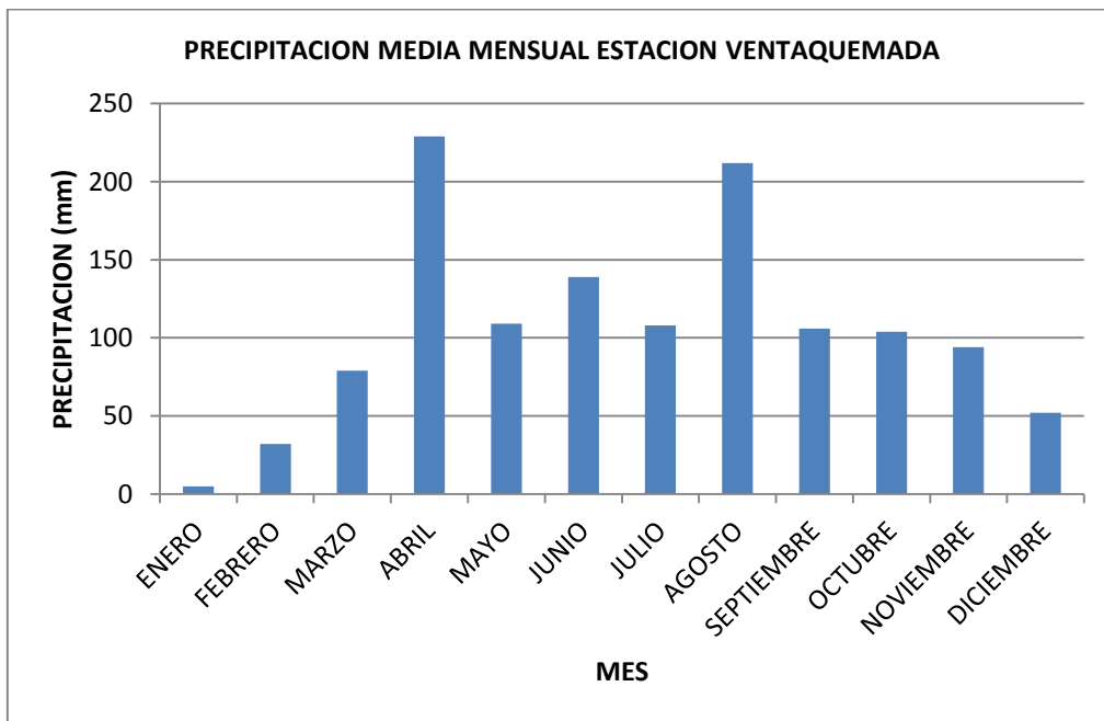
Figura .Precipitación media mensual estación Ventaquemada (1978)
