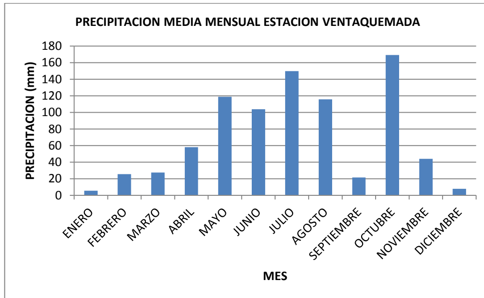
Figura .Precipitación media mensual estación Ventaquemada (1987)
