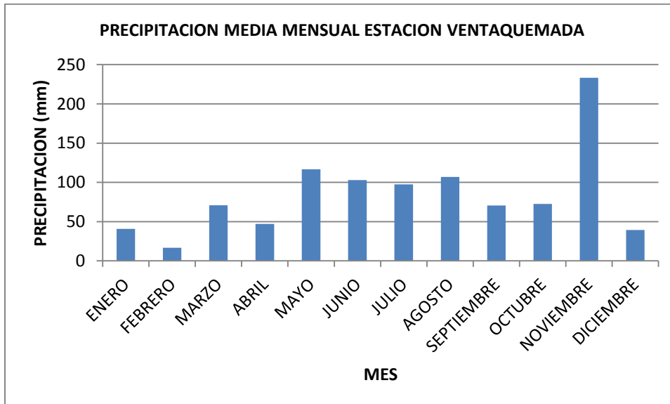
Figura .Precipitación media mensual estación Ventaquemada (2007)
