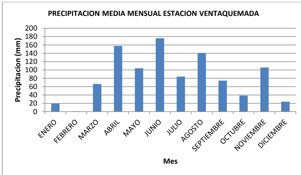
Figura .Precipitación media mensual Ventaquemada (1967)
