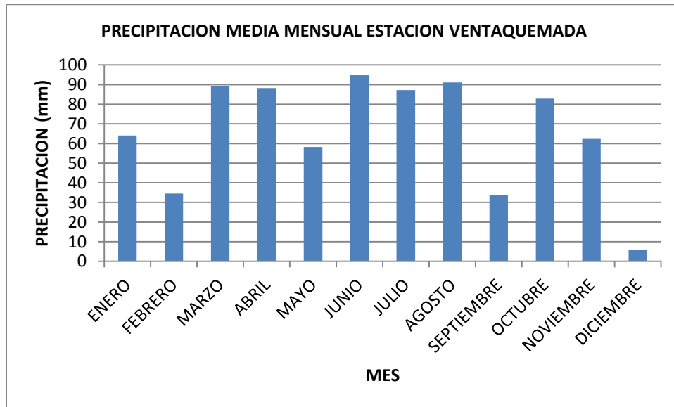
Figura .Precipitación media mensual estación Ventaquemada (2009)
