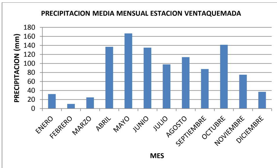
Figura .Precipitación media mensual estación Ventaquemada (2004)
