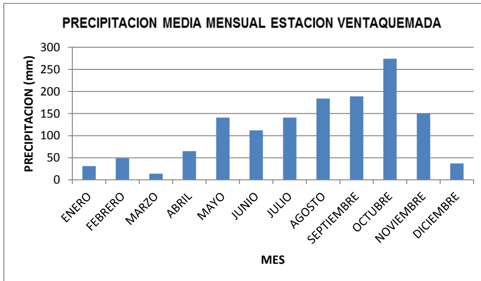
Figura .Precipitación media mensual estación ventaquemada (1970)
