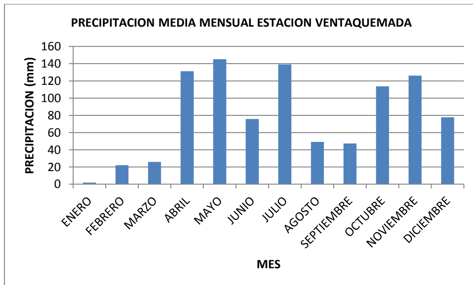
Figura .Precipitación media mensual estación Ventaquemada (2010)
