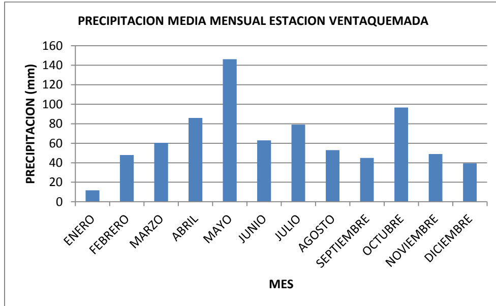
Figura .Precipitación media mensual estación Ventaquemada (1990)
