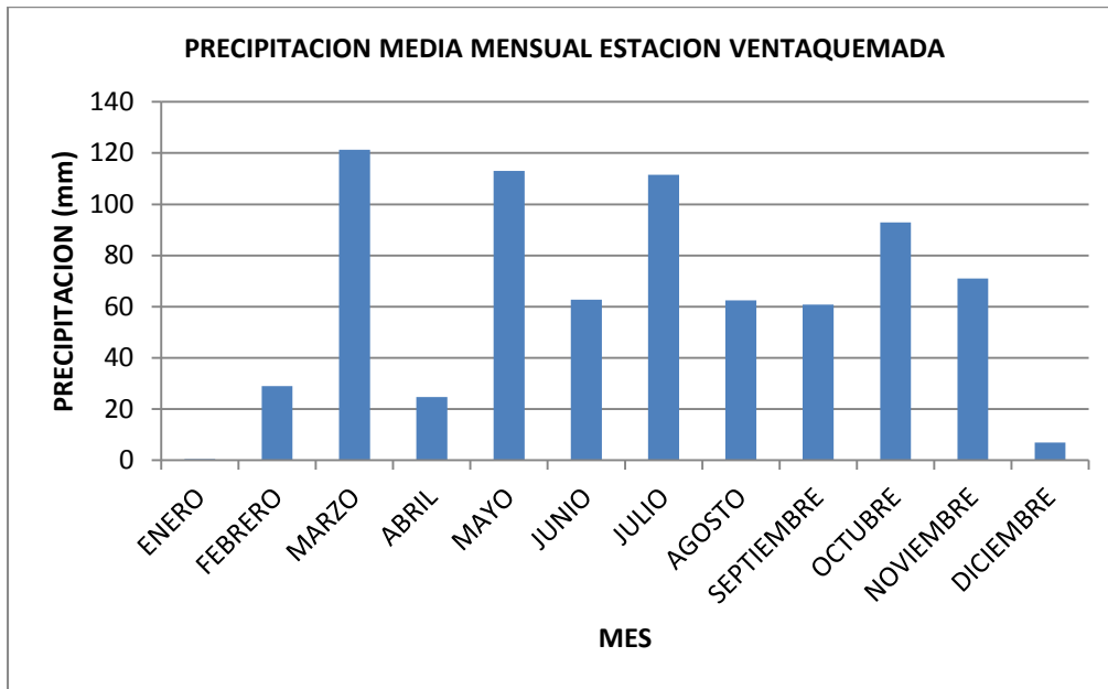
Figura .Precipitación media mensual estación Ventaquemada (1989)
