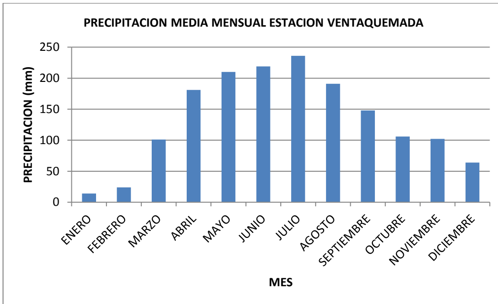
Figura .Precipitación media mensual estación Ventaquemada (1973)
