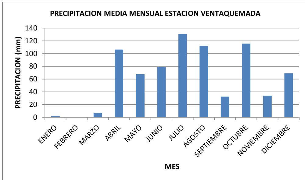
Figura .Precipitación media mensual estación Ventaquemada (1983)
