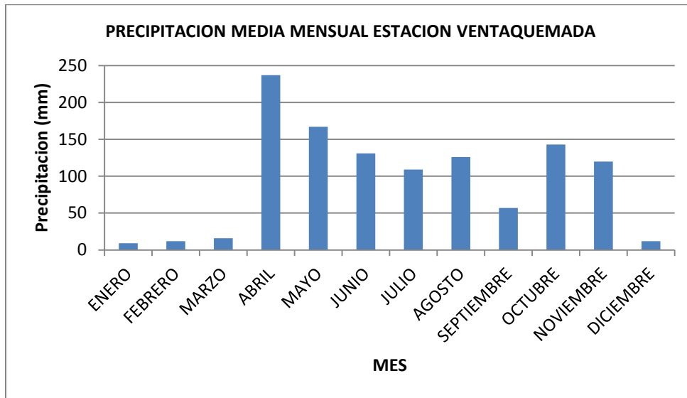
Figura .Precipitación media mensual estación Ventaquemada (1965)
