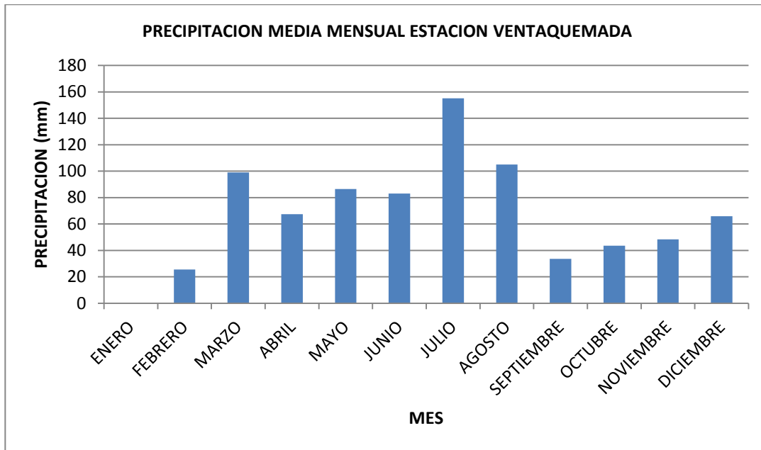
Figura .Precipitación media mensual estación Ventaquemada (1991)
