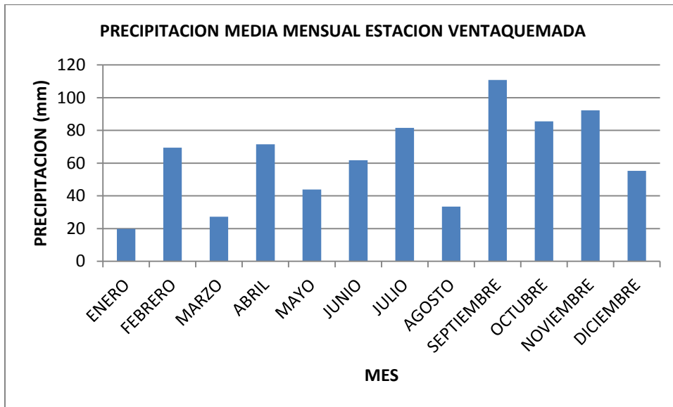
Figura .Precipitación media mensual estación Ventaquemada (1999)
