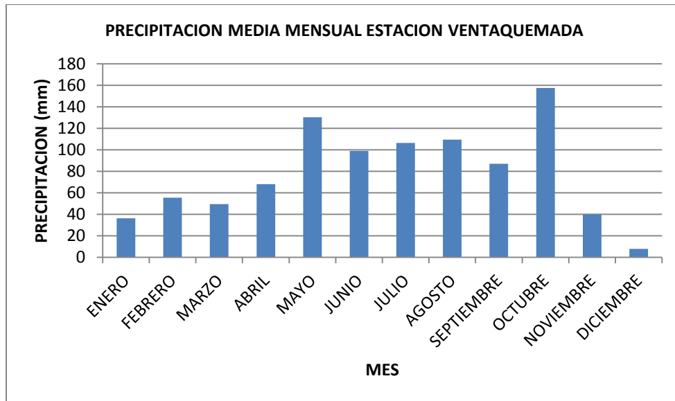
Figura .Precipitación media mensual estación Ventaquemada (1994)
