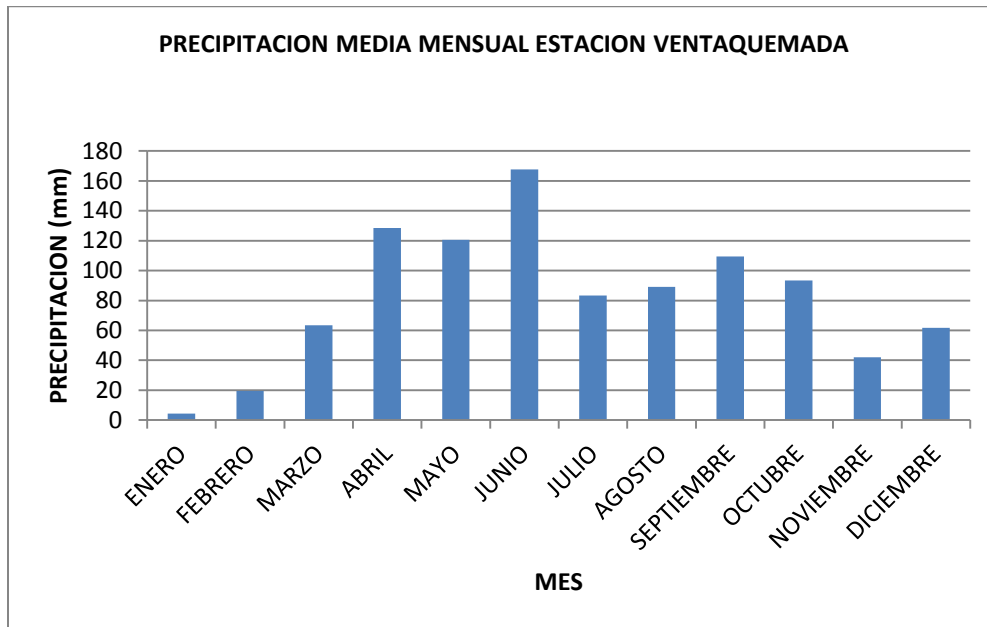
Figura .Precipitación media mensual estación Ventaquemada (1985)
