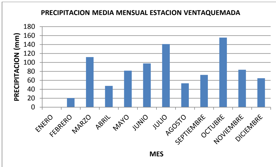
Figura .Precipitación media mensual estación Ventaquemada (2003)
