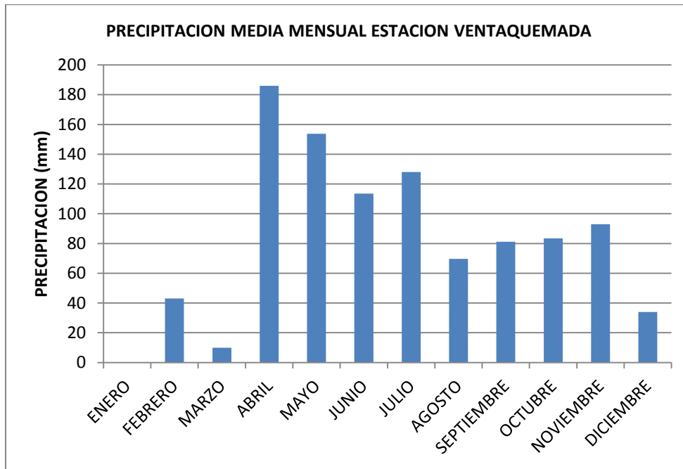
Figura .Precipitación media mensual estación Ventaquemada (1981)
