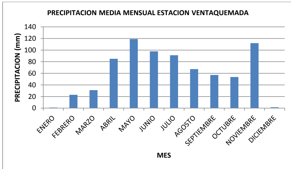
Figura .Precipitación media mensual estación Ventaquemada (1993)
