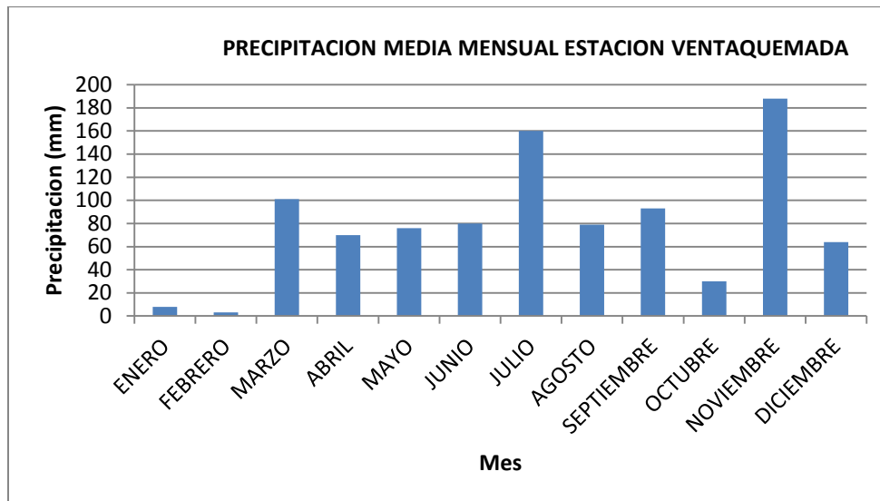
Figura .Precipitación media mensual estación Ventaquemada (1966)
