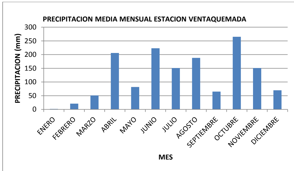
Figura .Precipitación media mensual estación Ventaquemada (1979)
