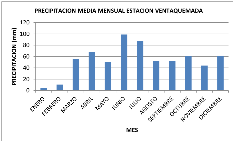
Figura .Precipitación media mensual estación Ventaquemada (1995)
