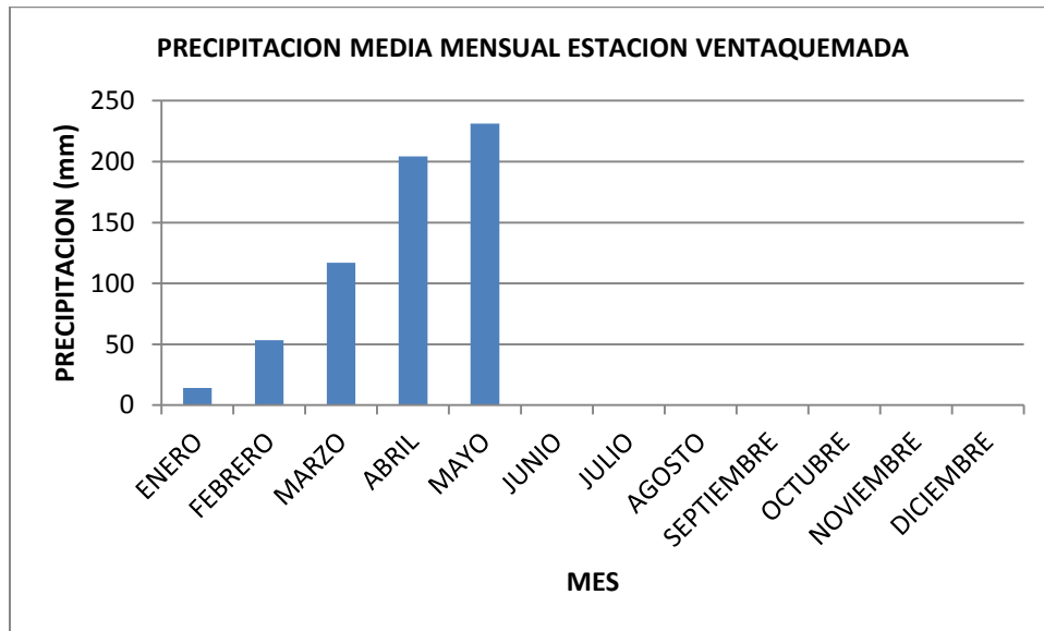
Figura .Precipitación media mensual estación Ventaquemada (2011)
