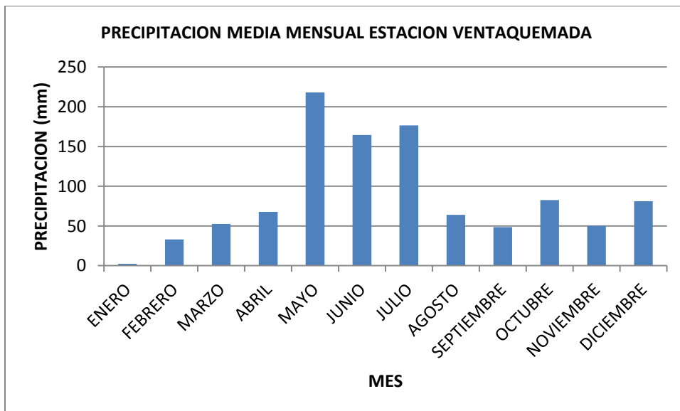
Figura .Precipitación media mensual estación Ventaquemada (1998)
