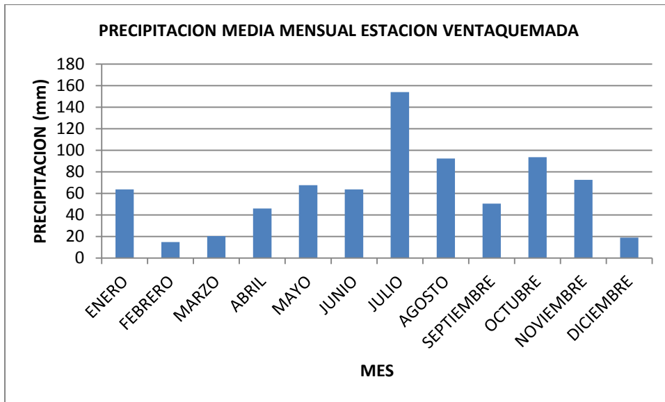
Figura .Precipitación media mensual estación Ventaquemada (1997)
