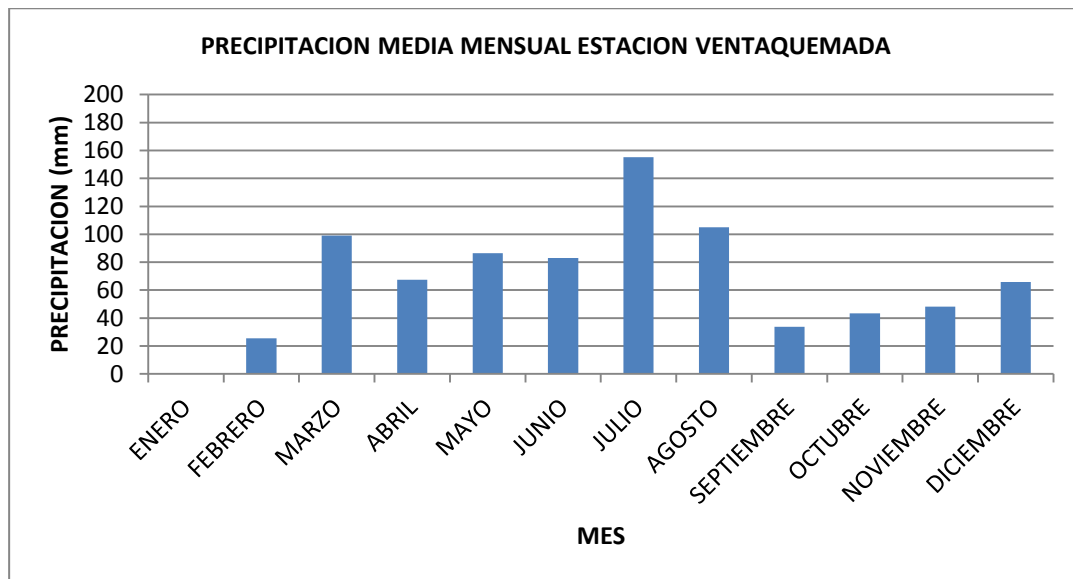
Figura .Precipitación media mensual estación Ventaquemada (1992)
