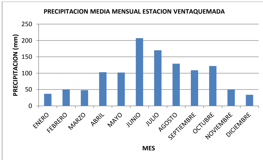
Figura .Precipitación media mensual estación Ventaquemada (1980)
