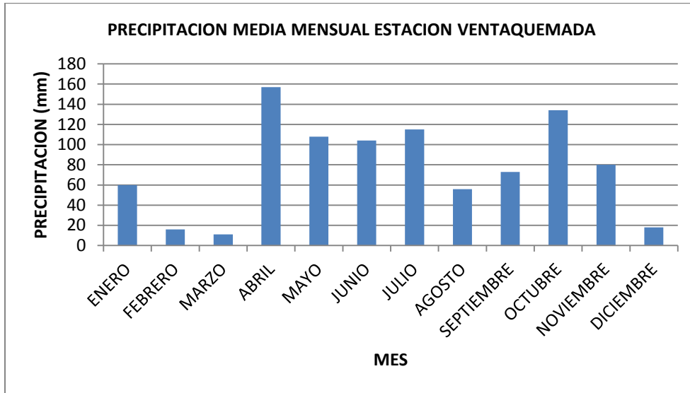
Figura .Precipitación media mensual estación Ventaquemada (1969)
