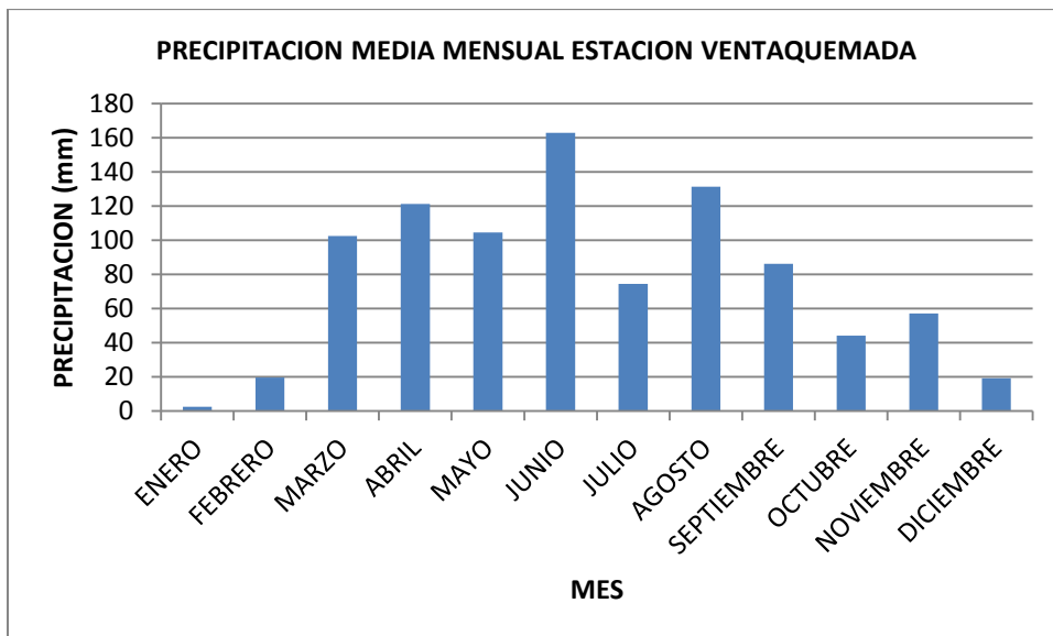
Figura .Precipitación media mensual estación Ventaquemada (2002)
