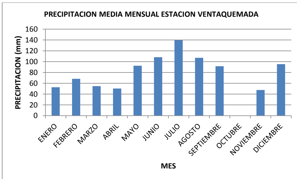
Figura .Precipitación media mensual estación Ventaquemada (1996)
