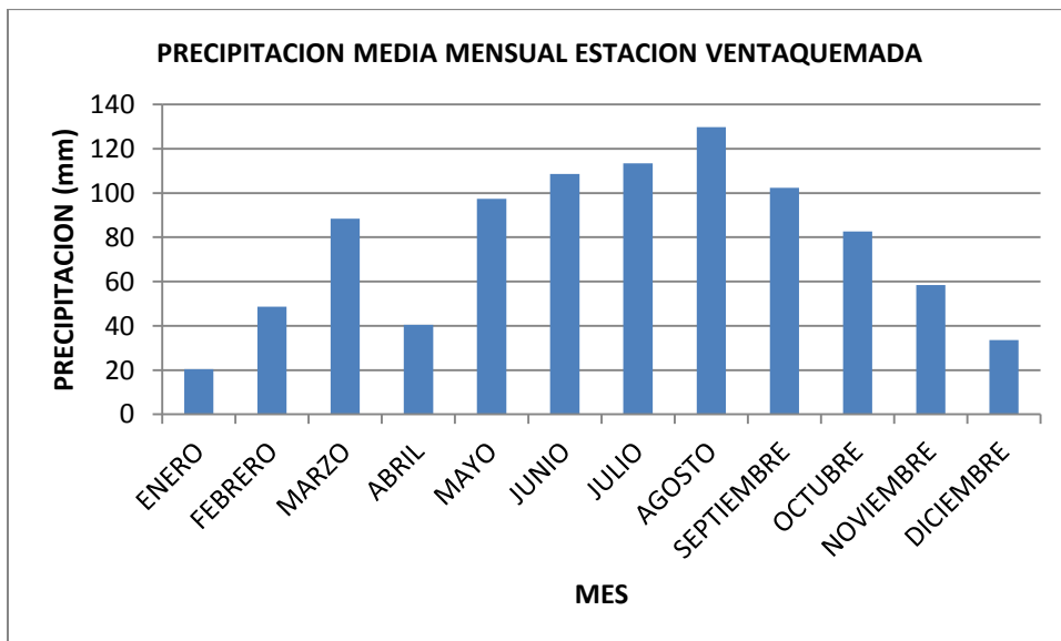
Figura .Precipitación media mensual estación Ventaquemada (2000)
