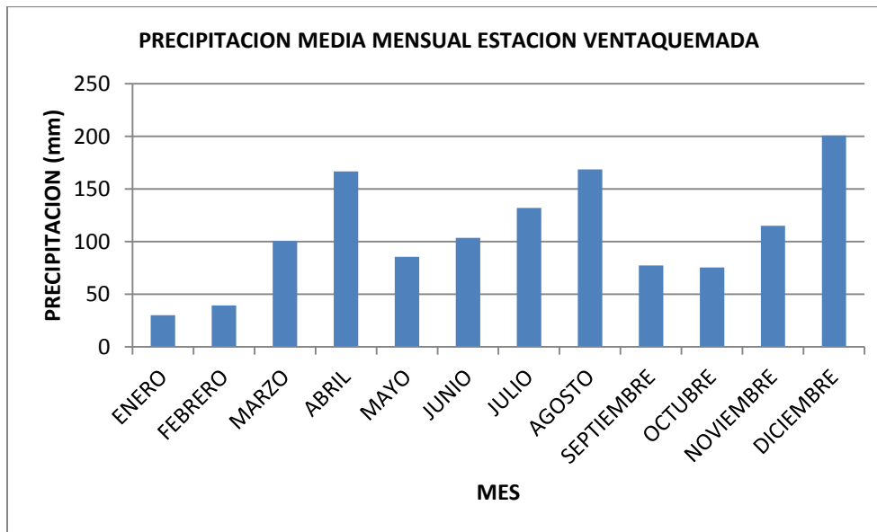
Figura .Precipitación media mensual estación Ventaquemada (1982)
