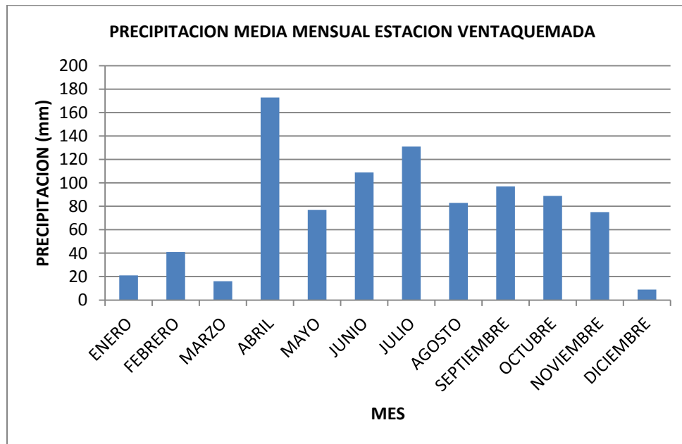
Figura .Precipitación media mensual estación Ventaquemada (1968)
