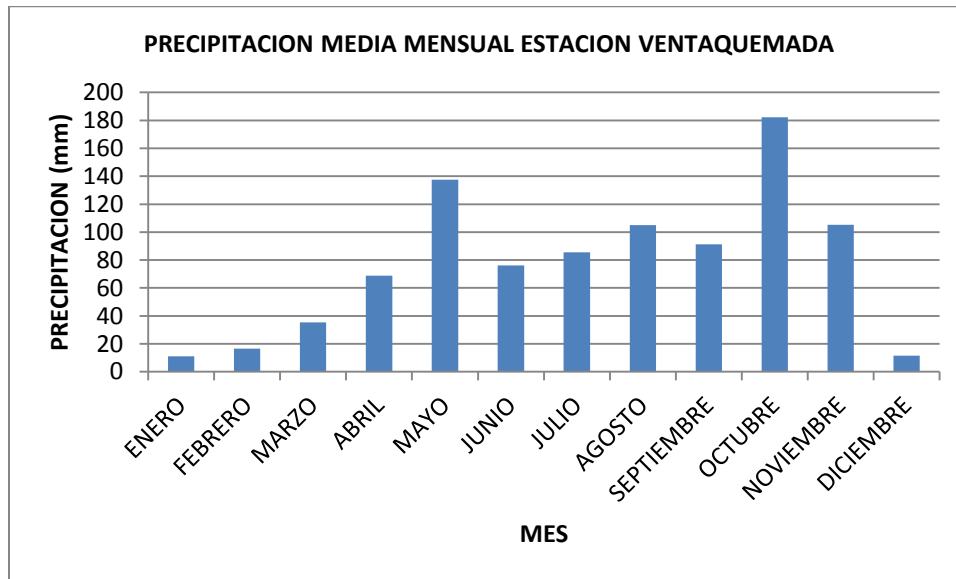
Figura .Precipitación media mensual estación Ventaquemada (2005)
