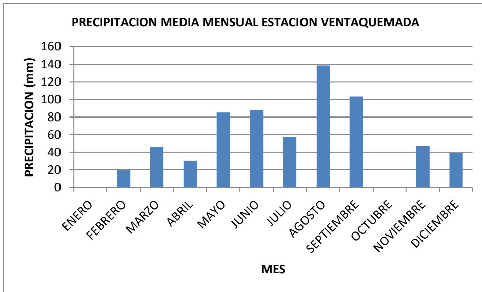
Figura .Precipitación media mensual estación Ventaquemada (2001)
