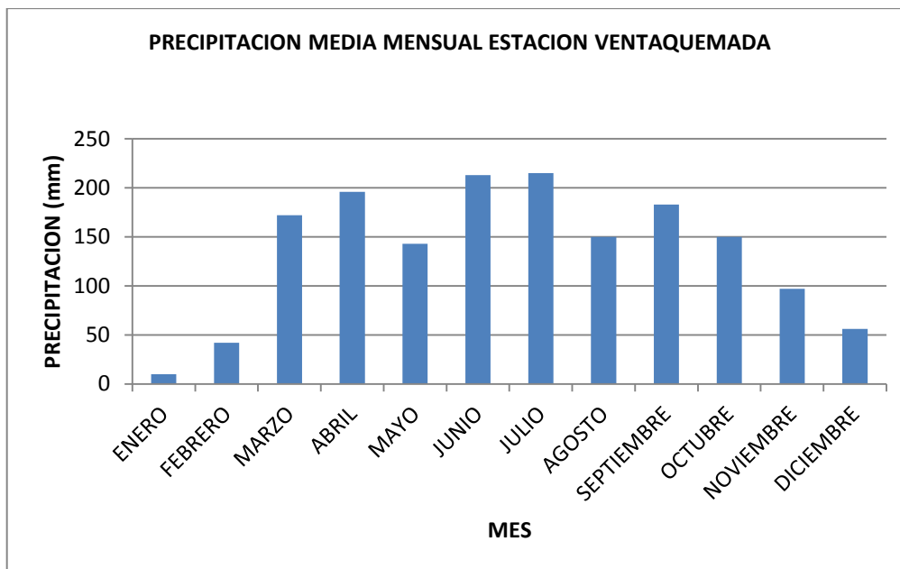
Figura .Precipitación media mensual estación Ventaquemada (1976)
