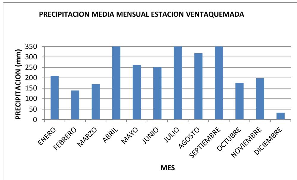
Figura .Precipitación media mensual estación Ventaquemada (1972)
