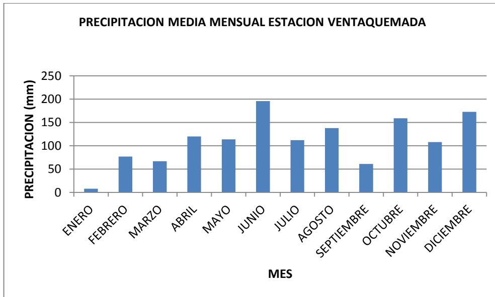
Figura .Precipitación media mensual estación Ventaquemada (1975)
