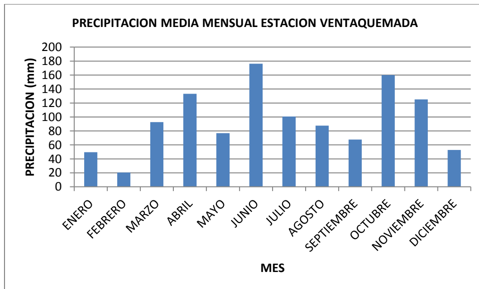
Figura .Precipitación media mensual estación Ventaquemada (2006)
