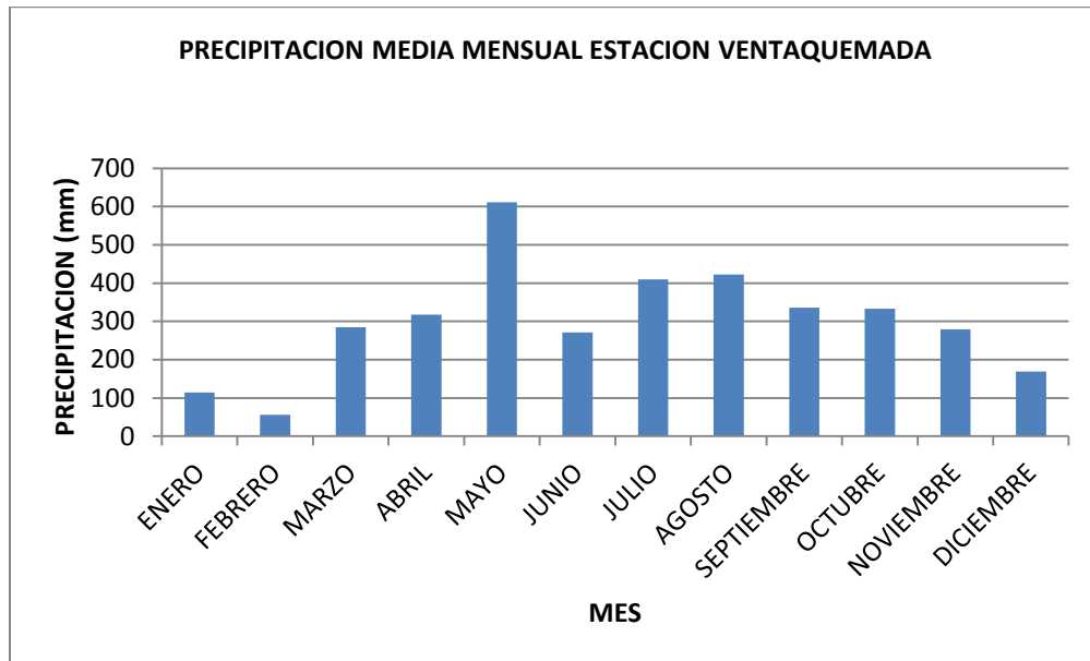
Figura .Precipitación media mensual estación Ventaquemada (1971)
