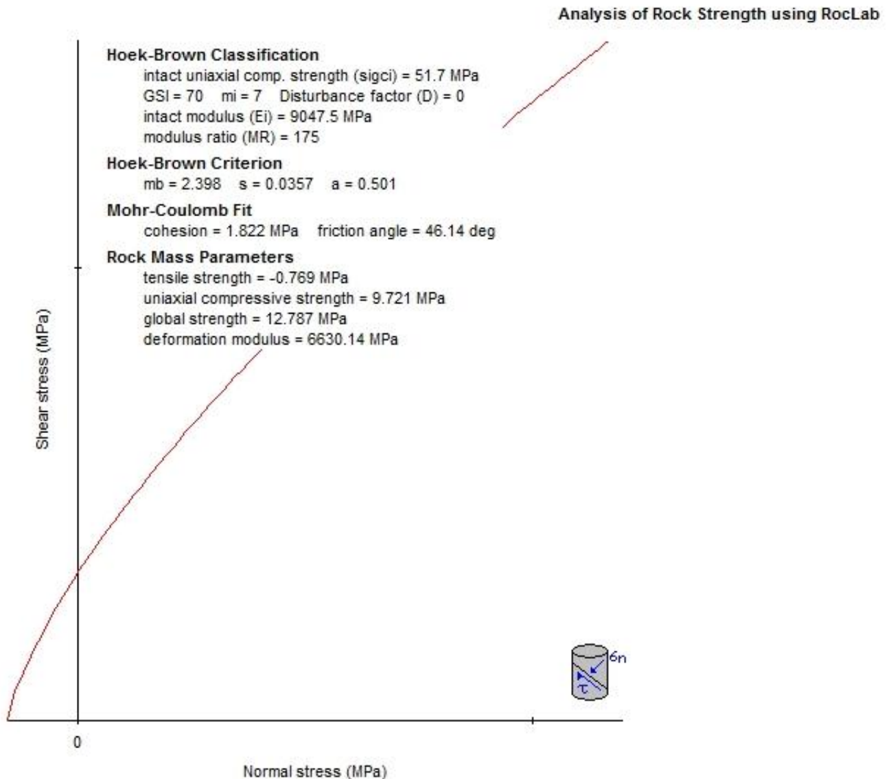
Figura 3. Salida gráfica del software RocLab 1.0 para la caracterización mecánica de la roca.
