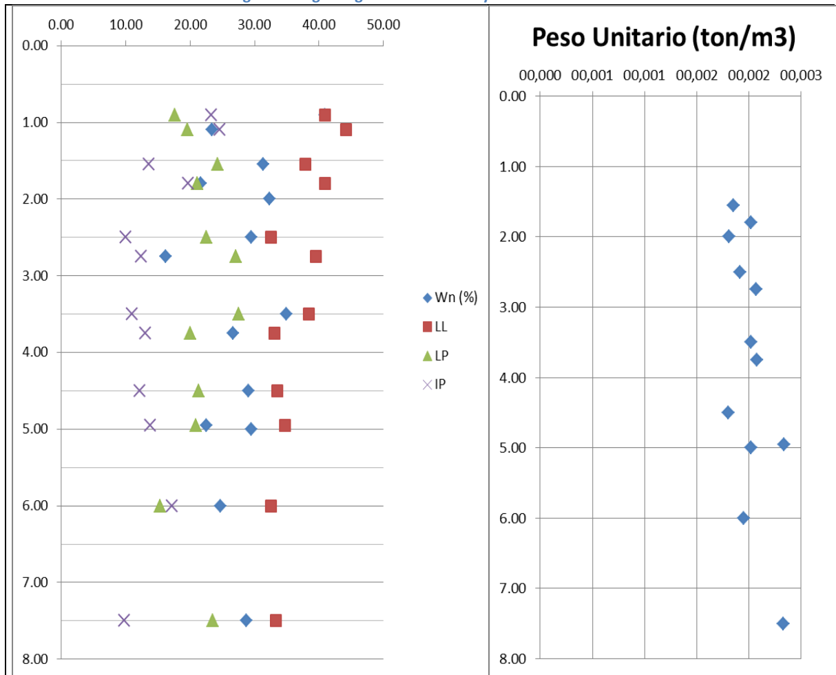
Figura 1. Registro gráfico de los ensayos de laboratorio.
