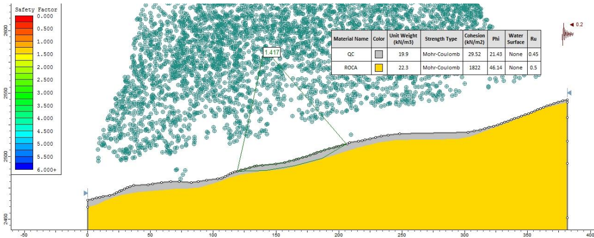
Figura 6. Distribución de los FS para el escenario actual en la condición extrema del Perfil C.
