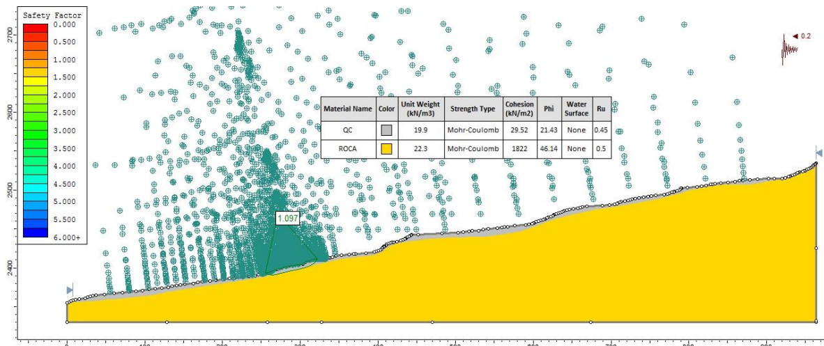
Figura 5. Distribución de los FS para el escenario actual en la condición extrema del Perfil B.
