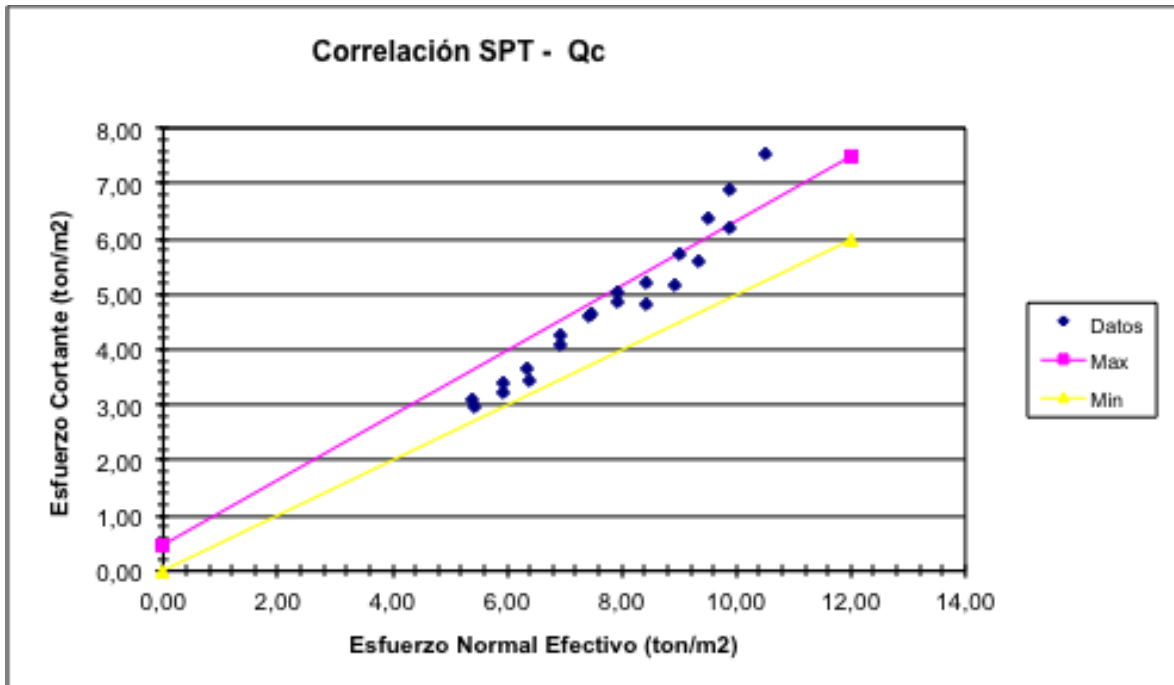
Figura 2. Análisis de los parámetros de resistencia a partir del SPT.
