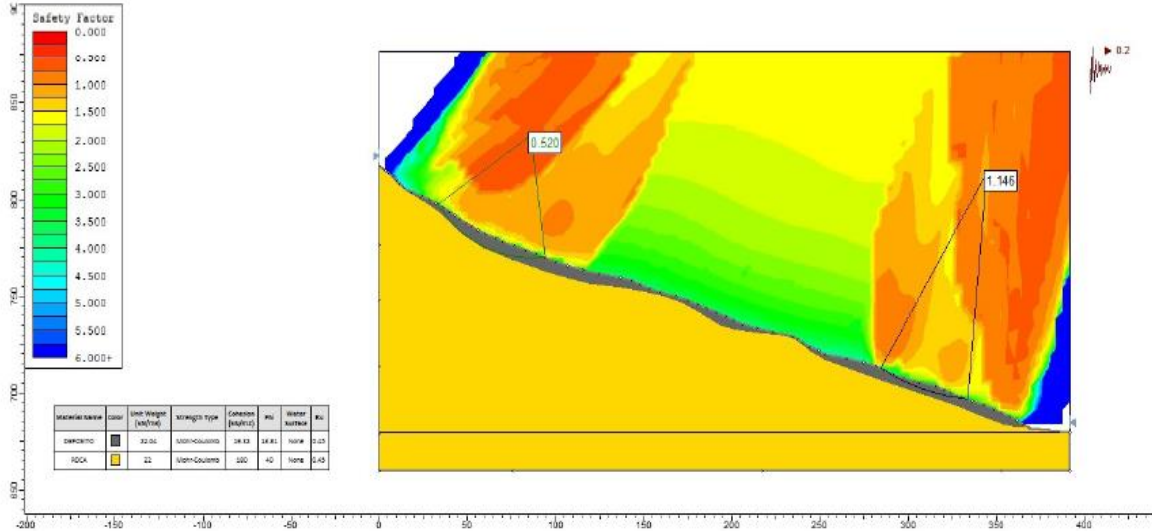
Figura 7. Distribución de los FS para el escenario actual en la condición extrema del Perfil BB Rotacional.
