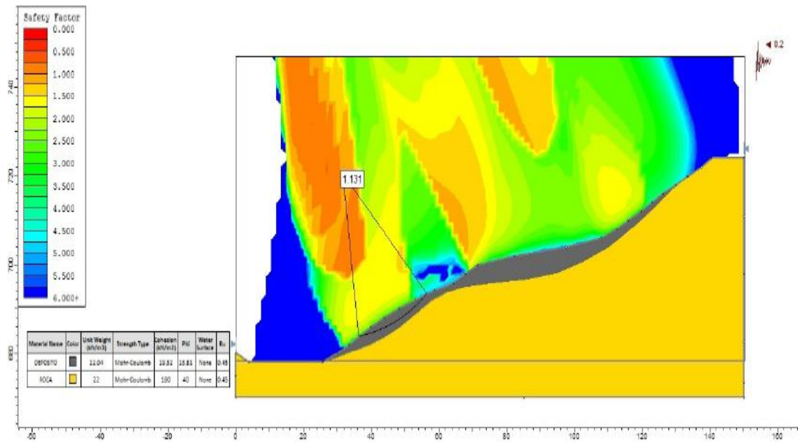
Figura 6. Distribución de los FS para el escenario actual en la condición extrema del Perfil AA Rotacional.
