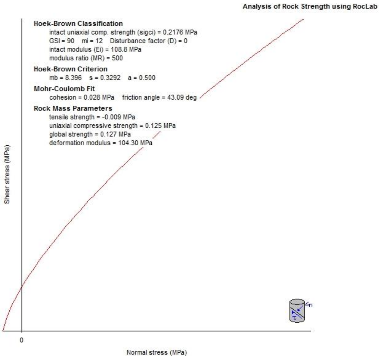
Figura 2. Salida gráfica del software RocLab 1.0 para la caracterización mecánica de la roca.
