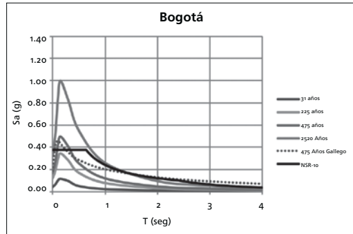
Figura 16. Espectros de amenaza uniforme para diferentes períodos de retorno Bogotá
