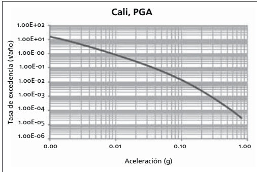
Figura 17. Curva de amenaza PGA Cali
