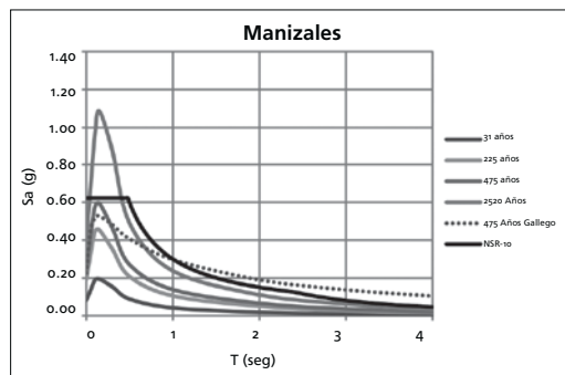
Figura 20. Espectros de amenaza uniforme para diferentes períodos de retorno Manizales
