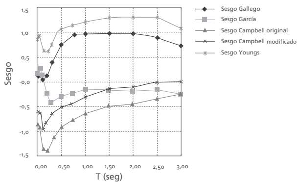
Figura 9. Comparación sesgos zona de Benioff
