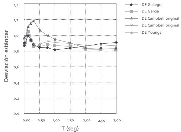
Figura 10. Comparación desviaciones estándar zona de Benioff
