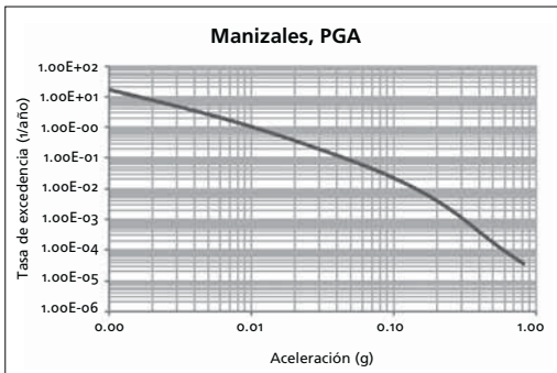
Figura 19. Curva de amenaza PGA Manizales
