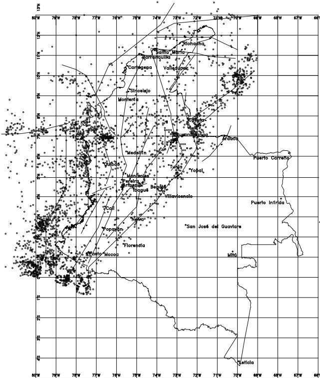
Figura 3. Eventos asignados a fuentes corticales
