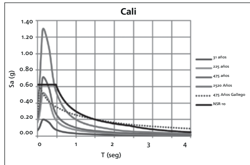
Figura 18. Espectros de amenaza uniforme para diferentes períodos de retorno Cali
