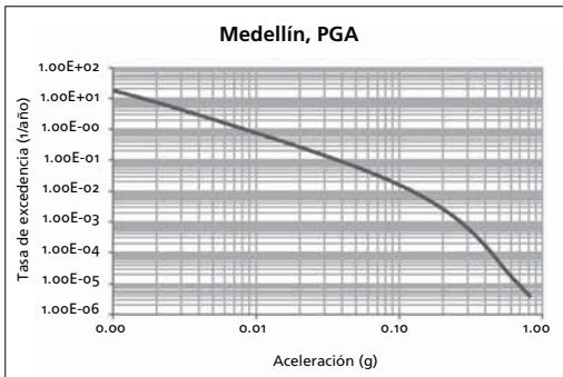
Figura 21. Curva de amenaza PGA Medellín
