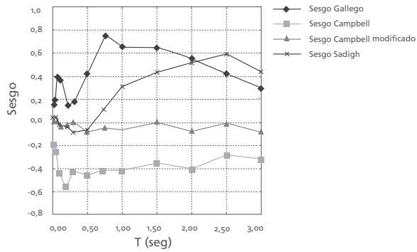
Figura 5. Comparación sesgos zona cortical
