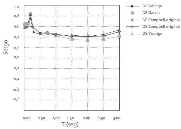
Figura 8. Comparación desviaciones estándar zona subducción
