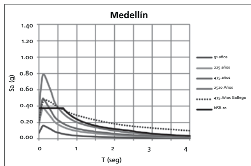
Figura 22. Espectros de amenaza uniforme para diferentes períodos de retorno Medellín
