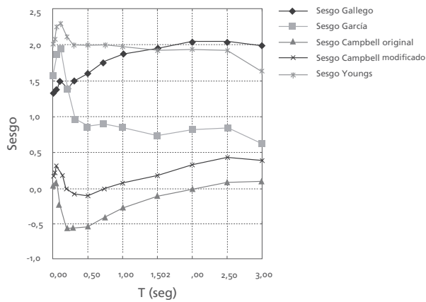
Figura 7. Comparación sesgos zona subducción
