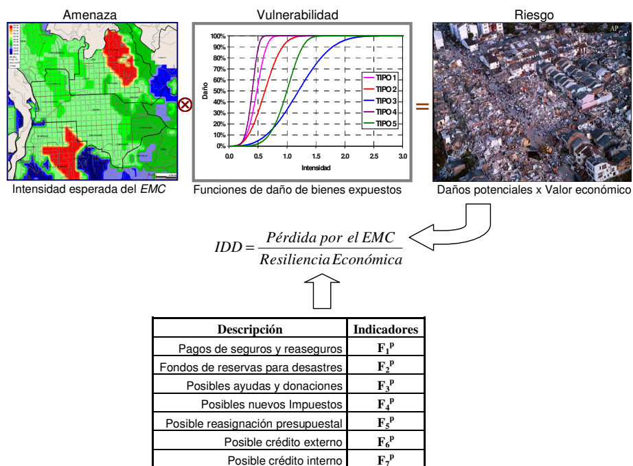
Figura 1. Diagrama para el cálculo del IDD
