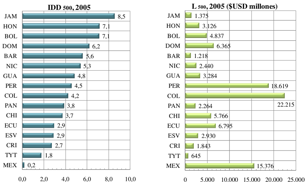
Figura 3. IDD y pérdida máxima probable en 500 años
