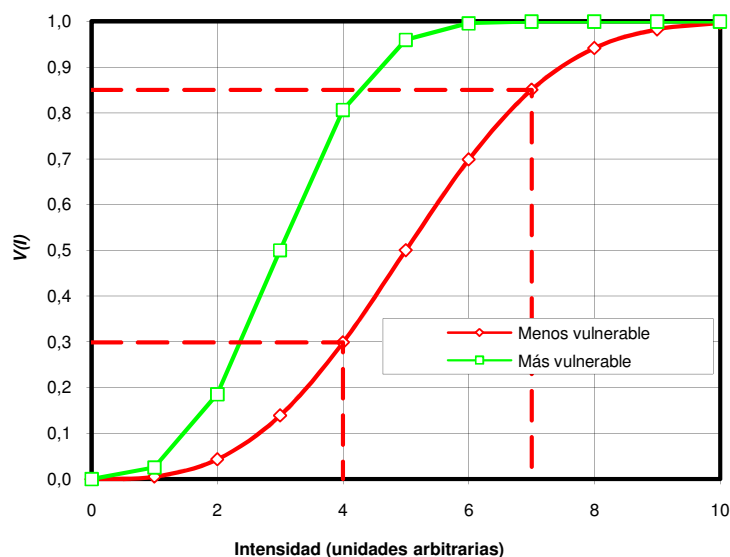
Figura 2. Representación de las funciones de vulnerabilidad
