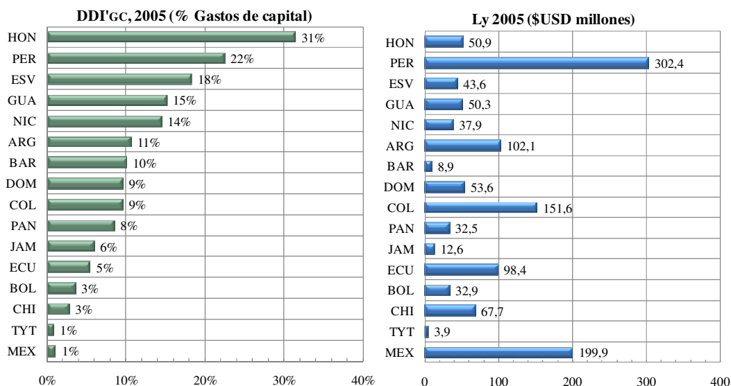
Figura 4. IDD'_{GC} y pérdida anual esperada
