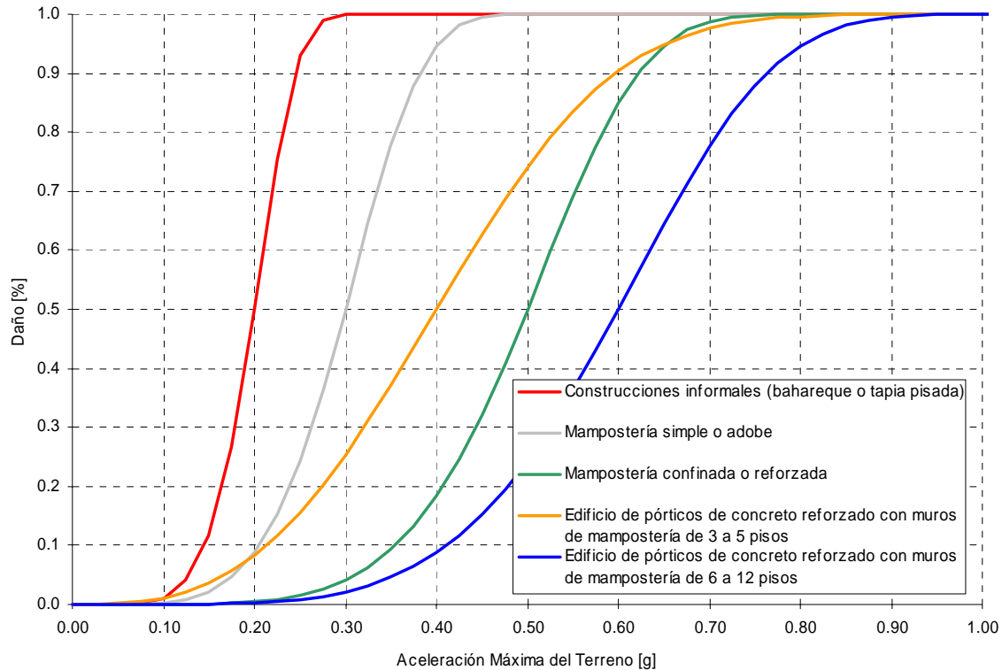
Figura 5-4 Funciones de vulnerabilidad representativas de los tipos constructivos en Colombia
