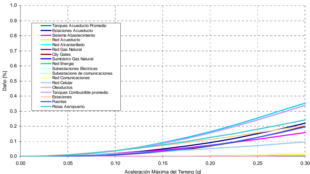
Figura 5-6 Funciones de vulnerabilidad de componentes de infraestructura
