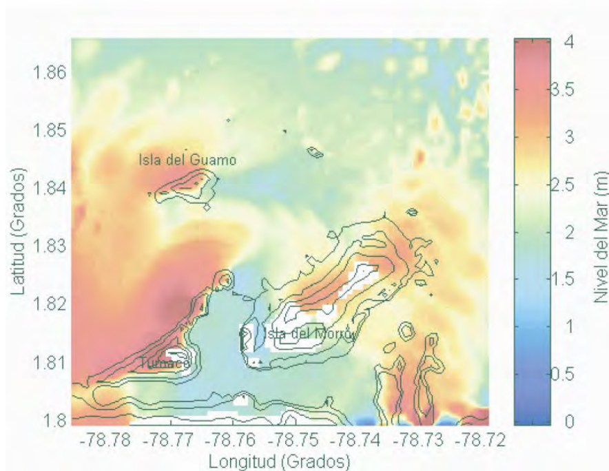
Figura 2-17 Mapa de inundación del área de Tumaco para el tsunami de 1979
