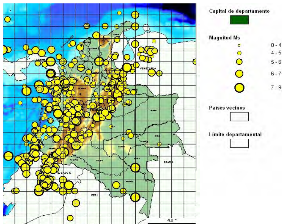
Figura 2-7 Mapa de grandes terremotos de Colombia 1566-1999
