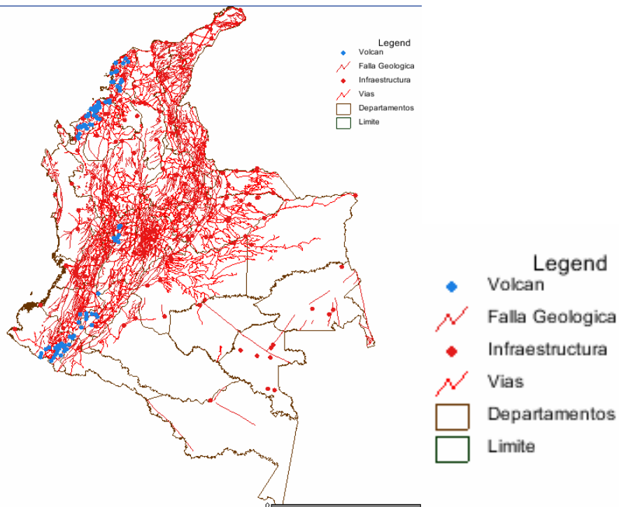
Figura 2-20 Distribución de volcanes, fallas geológicas, vías e infraestructura
