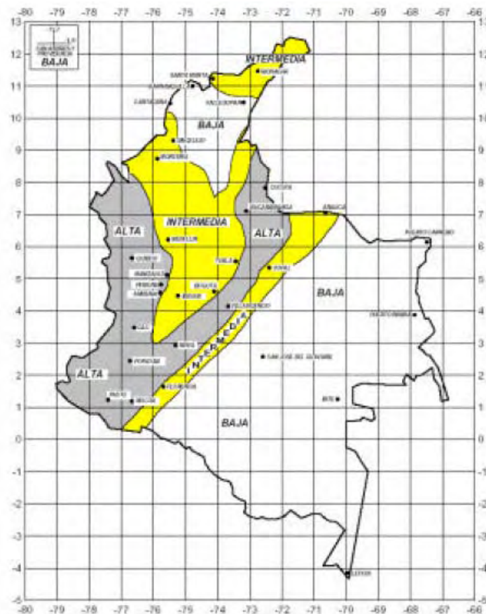
Figura 2-9 Mapa de amenaza sísmica de Colombia (NSR 98)
