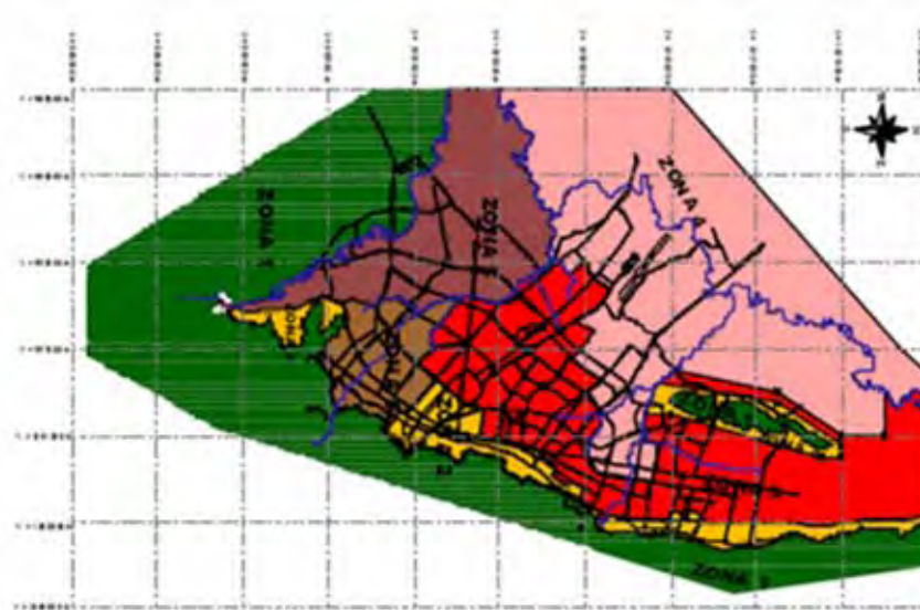
Figura 2-11 Microzonificación sísmica de Medellín
