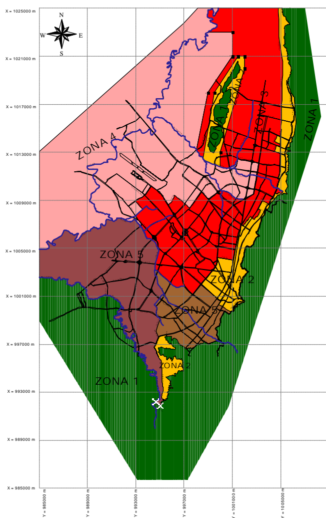
Figura 5-3 Microzonificación sísmica de Bogotá, Uniandes (1997)
