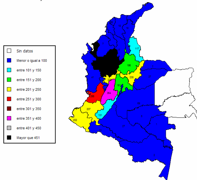
Figura A2-14 Clasificación por deslizamientos asociados a causas hidrológicas
