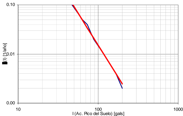
Figura 5-2 Modelo aproximado de la intensidad vs tasa de excedencia para la ciudad de Bogotá
