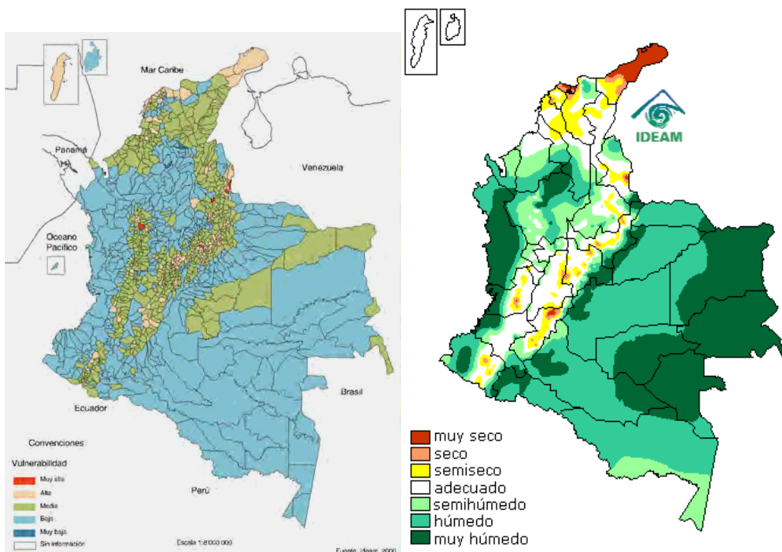
Figura 2-29 Índice de vulnerabilidad por escasez hídrica Figura 2-30 Mapa de disponibilidad hídrica
