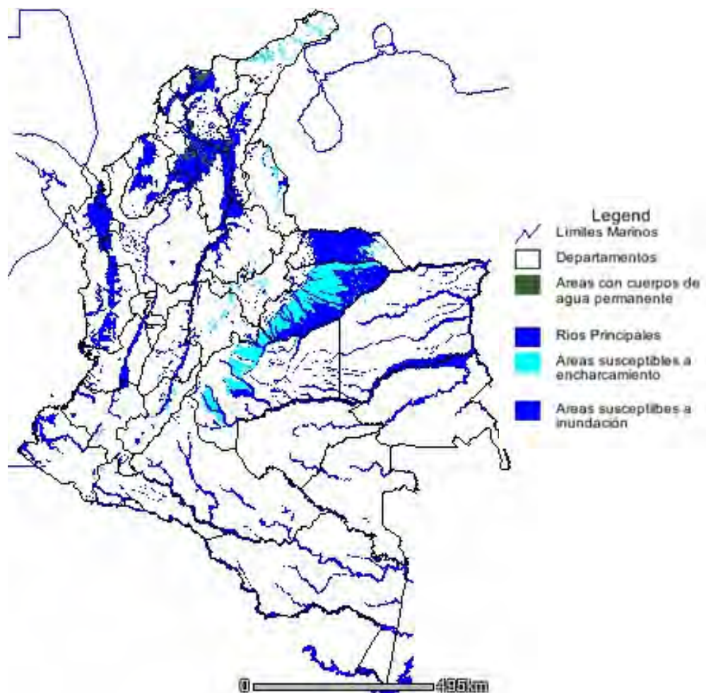
Figura 5-7 Mapa con zonas inundables, Colombia. (Fuente IDEAM)
