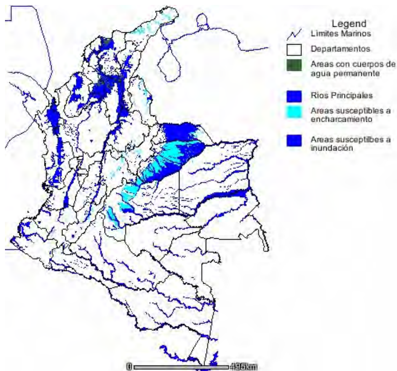
Figura 2-26 Mapa de zonas inundables. Fuente IDEAM
