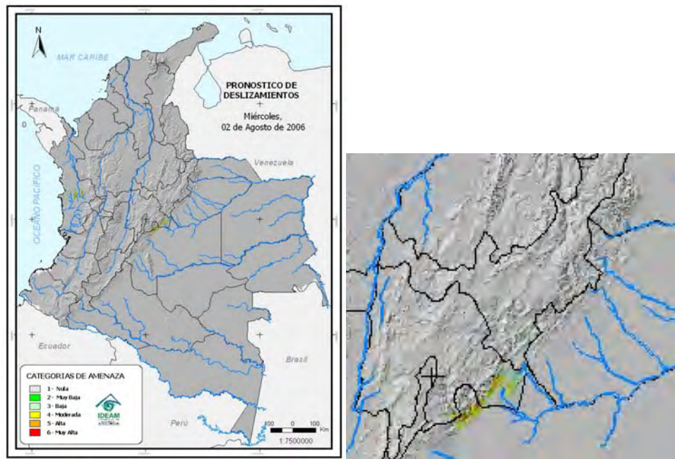
Figura 2-33 Pronósticos de zonas susceptibles a deslizamientos.
