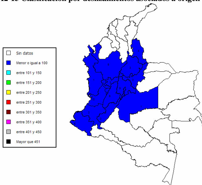
Figura A2-15 Clasificación por deslizamientos asociados a origen geológico
