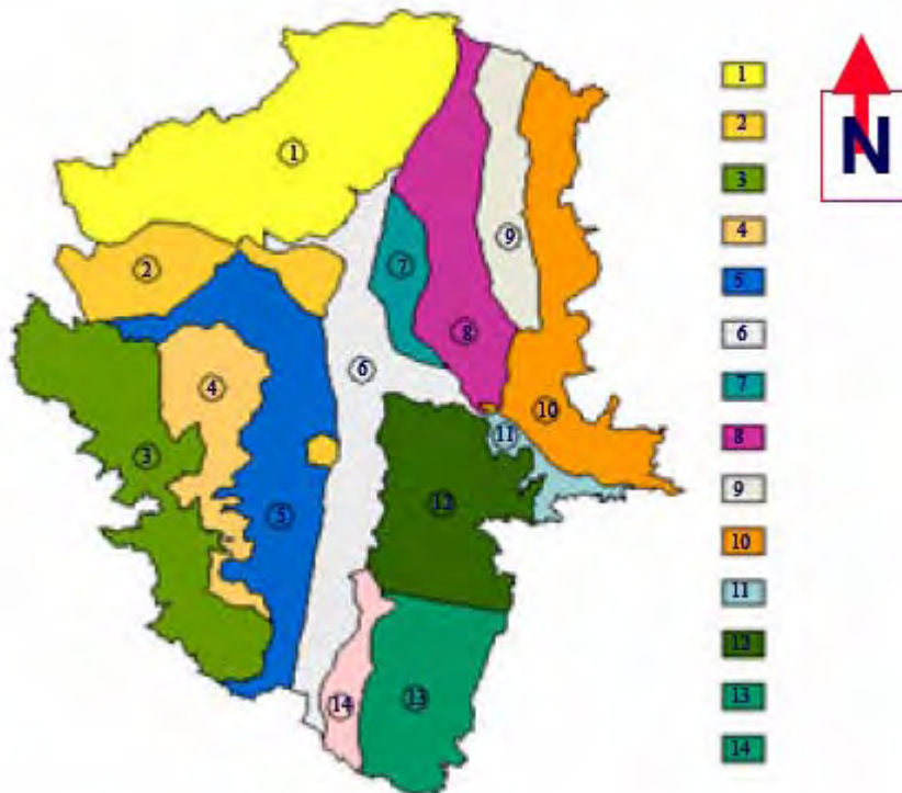
Figura 2-11 Microzonificación sísmica de Medellín
