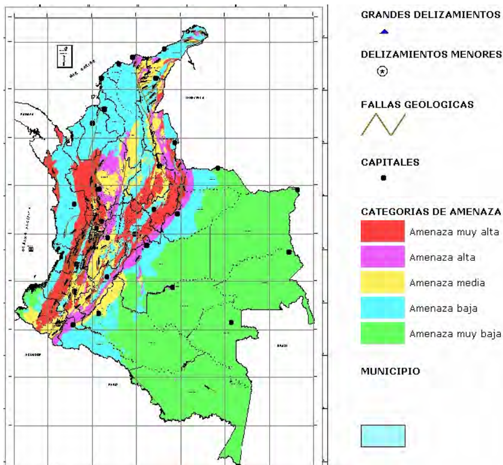
Figura 2-32 Mapa de categorías de amenaza relativa por movimientos de masa
