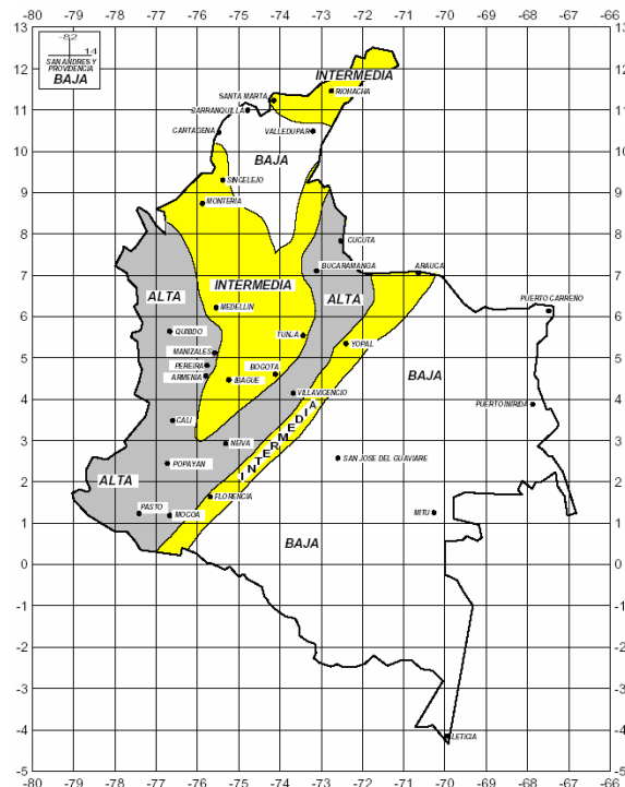
Figura 5-1 Mapa de Amenaza Sísmica. Fuente NSR 98 (AIS, 1998)
