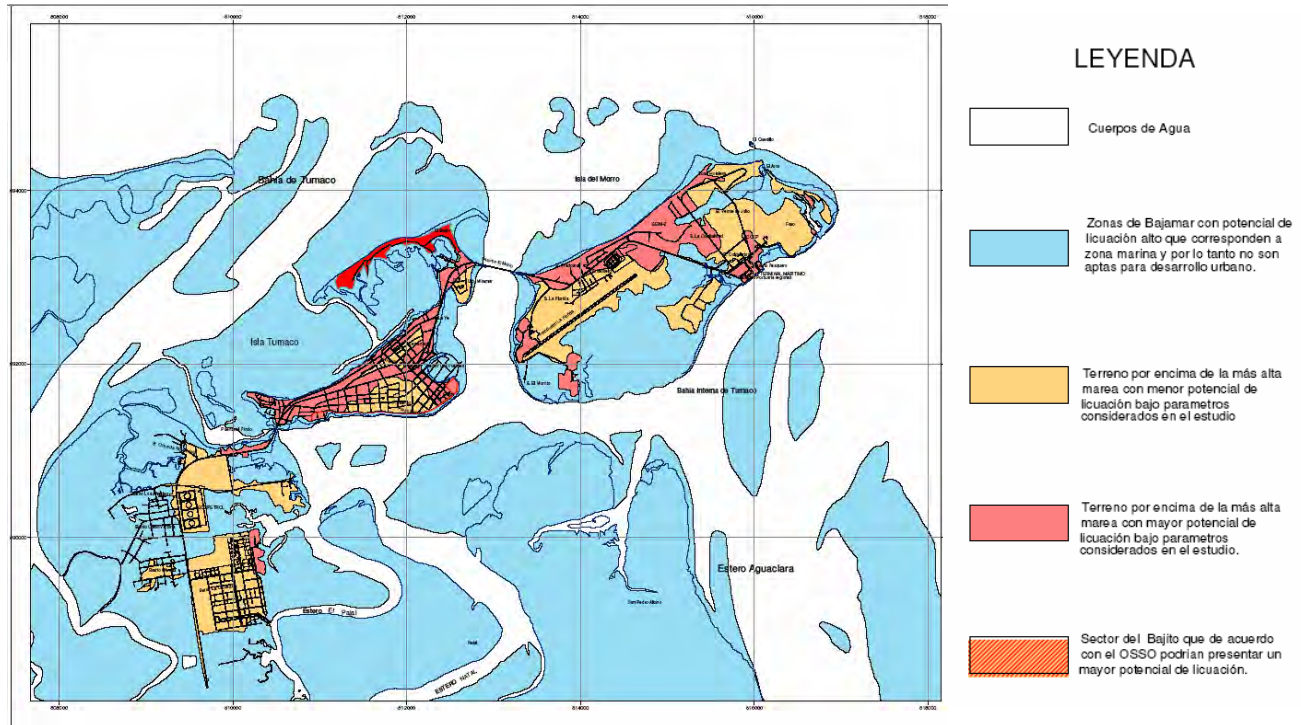
Figura 2-16 Mapa de zonificación geotécnica por licuación en el casco urbano de Tumaco
