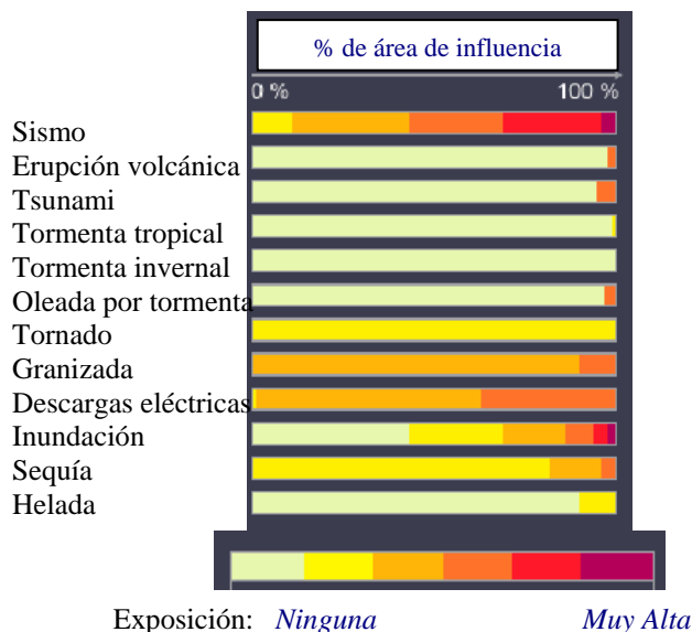
Figura 2-4 Área de influencia según el tipo de fenómeno, Fuente München RE
