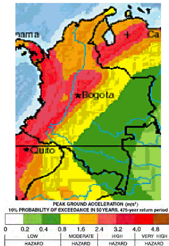
Figura 2-5 de Amenaza sísmica. Fuente “ http://www.seismo.ethz.ch/ ”
