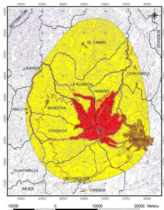
Figura 2-22 Mapa de amenaza del volcán Galeras
